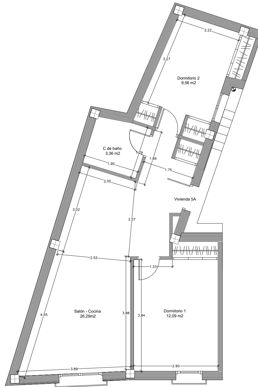
PLANTA DE COTAS Y SUPERFICIES
