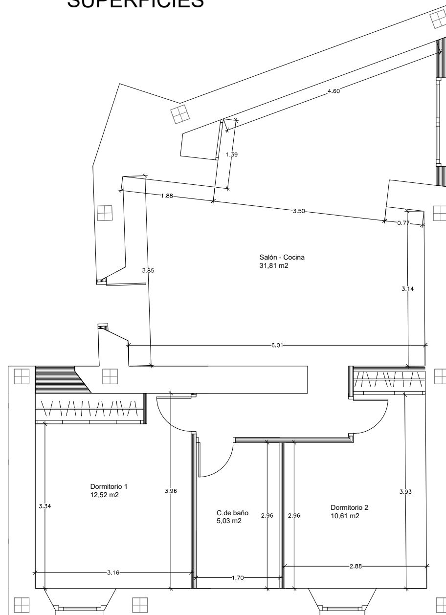
PLANTA DE COTAS Y SUPERFICIES
